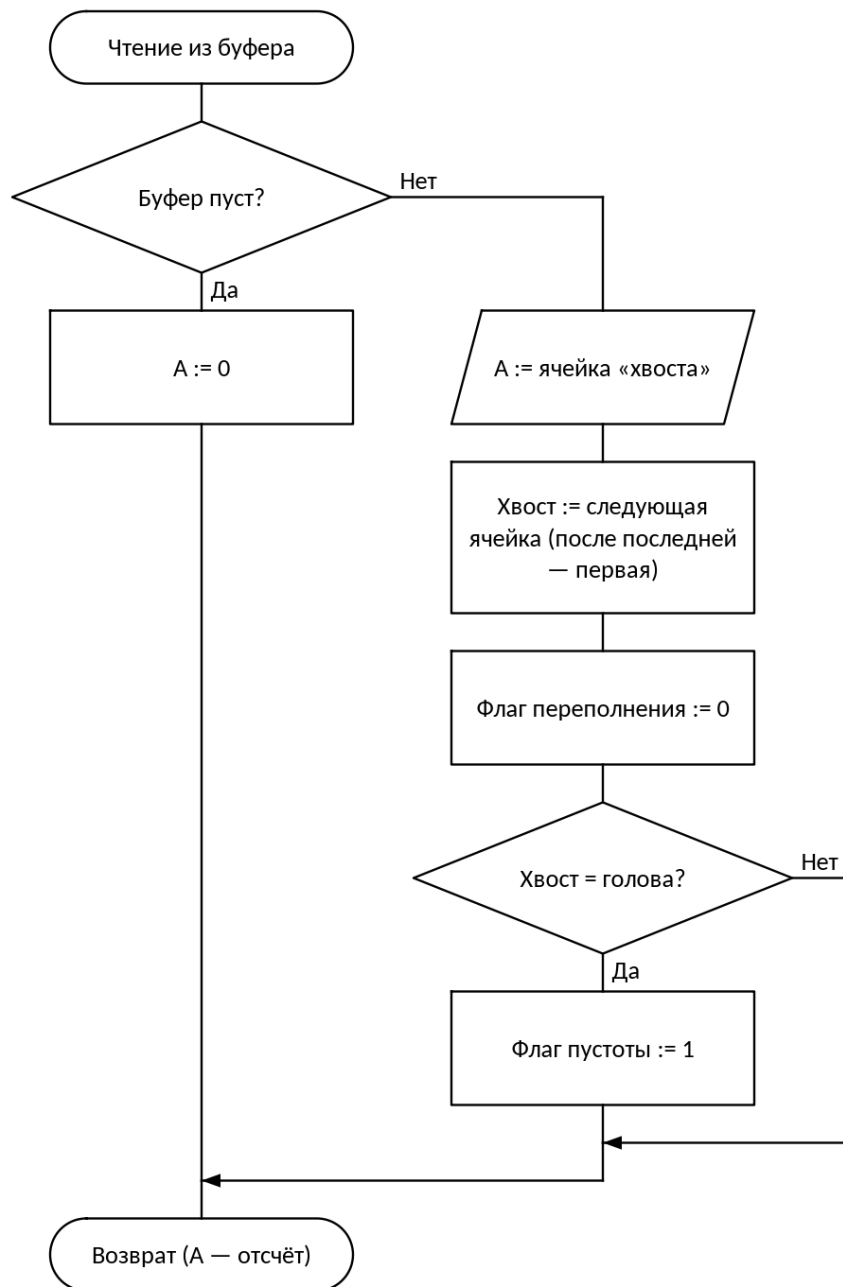
Рисунок 7 — Схема алгоритма: Чтение отсчёта из кольцевого буфера
