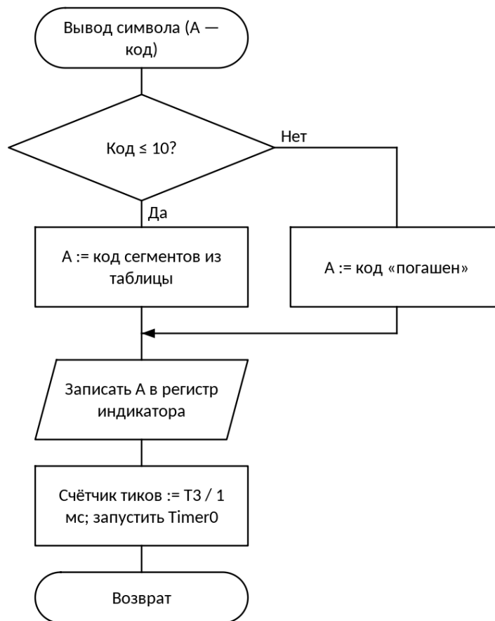
Рисунок 9 — Схема алгоритма: Вывод символа на индикатор
