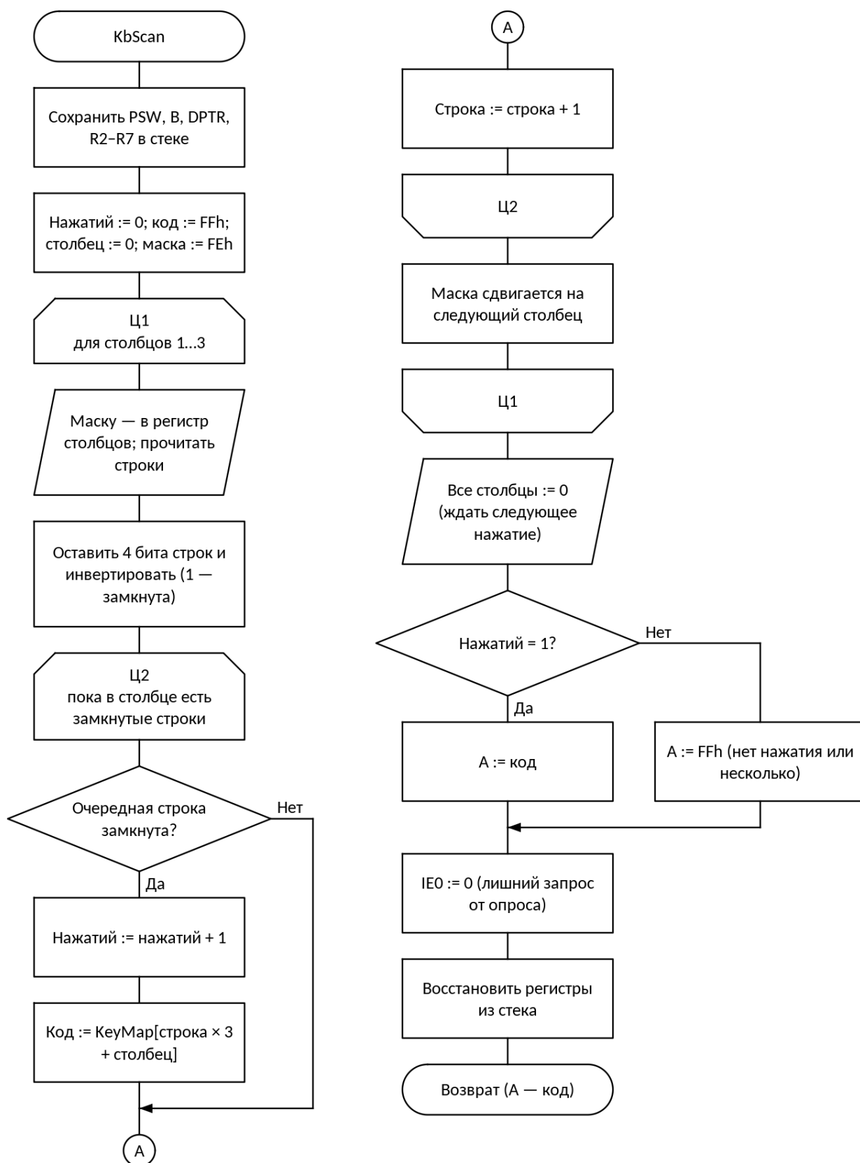
Рисунок 3 — Схема алгоритма: Опрос клавиатуры KbScan (обработчик INT0)
