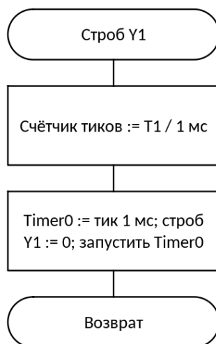
Рисунок 11 — Схема алгоритма: Начало строба Y1
