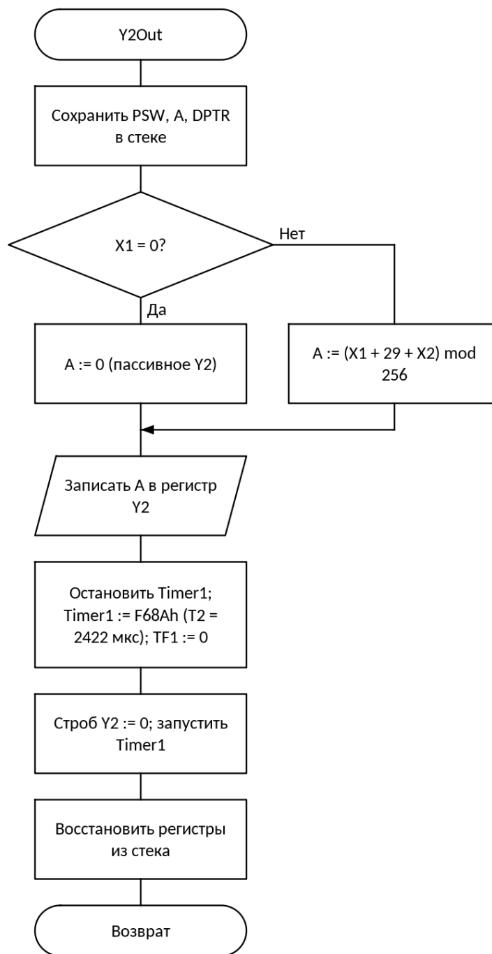
Рисунок 12 — Схема алгоритма: Расчёт и выдача сигнала Y2 (Y2Out)
