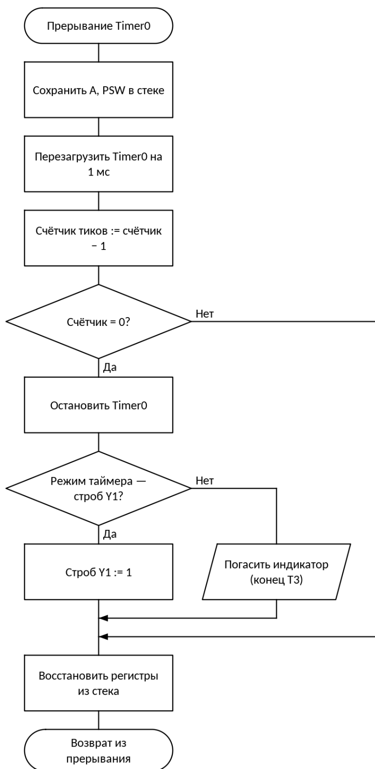
Рисунок 10 — Схема алгоритма: Обработчик прерывания Timer0: отсчёт T1 и T3
