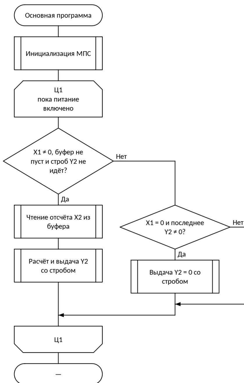
Рисунок 2 — Схема алгоритма: Основной цикл программы
