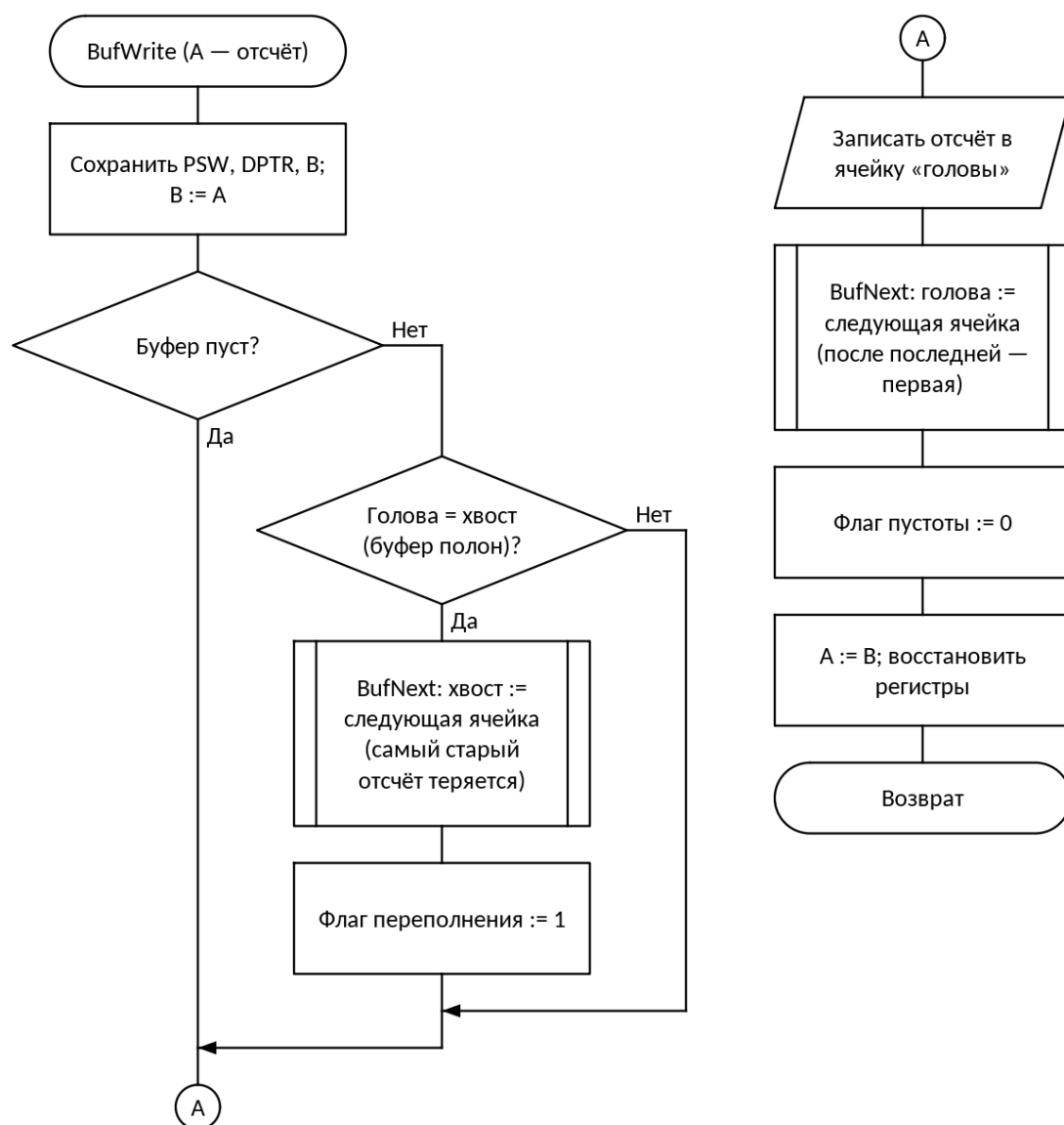
Рисунок 5 — Схема алгоритма: Запись отсчёта в кольцевой буфер BufWrite
