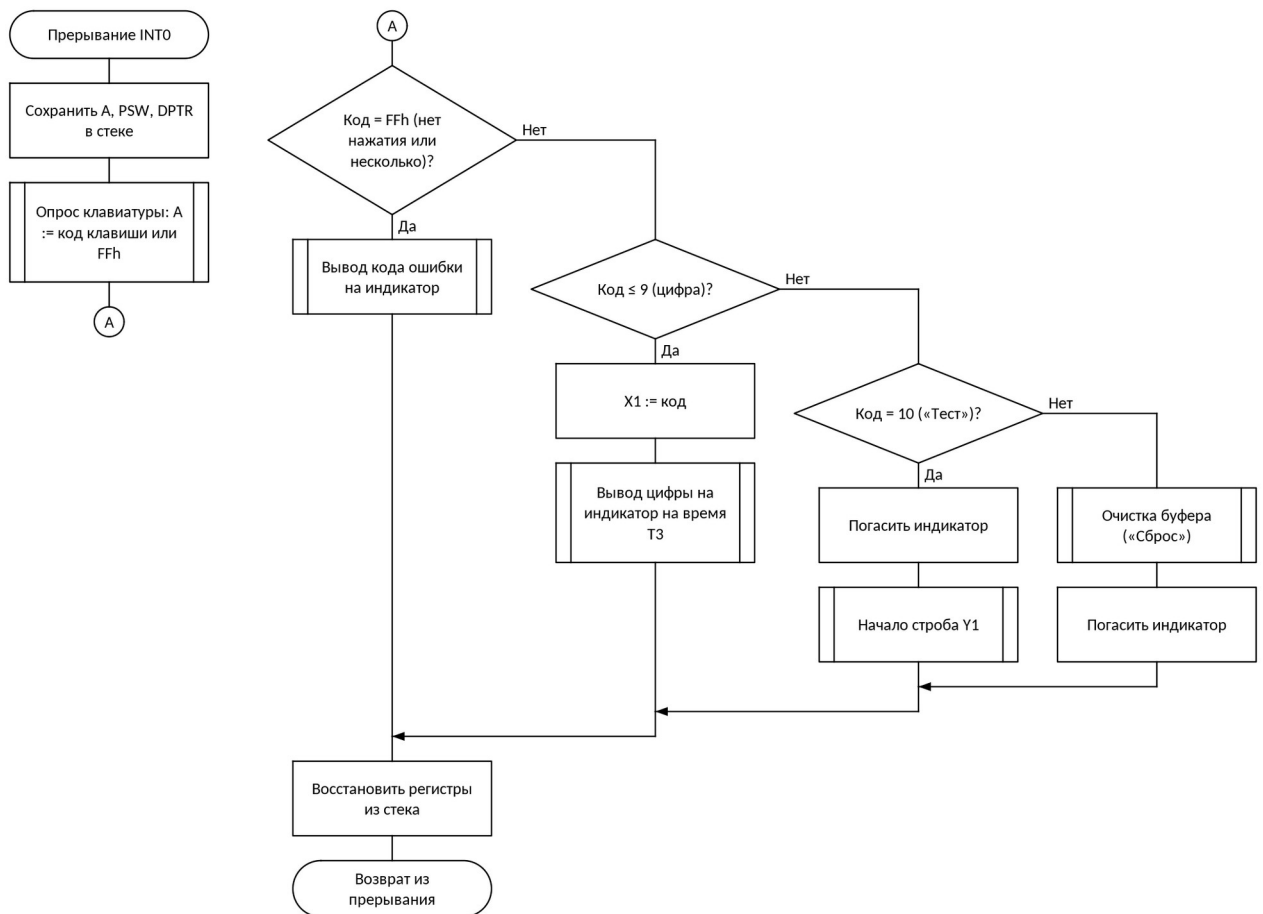
Рисунок 4 — Схема алгоритма: Обработчик прерывания INT0: реакция на клавишу
