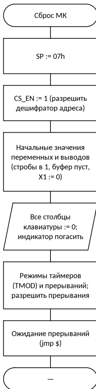
Рисунок 1 — Схема алгоритма: Инициализация МПС и основная программа
