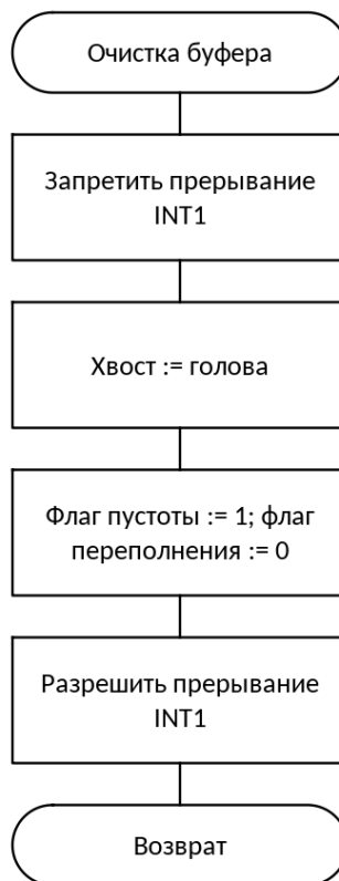
Рисунок 8 — Схема алгоритма: Очистка кольцевого буфера (клавиша «Сброс») Схема «Очистка кольцевого буфера (клавиша «Сброс»)» выполняется так: вход — «Очистка буфера»; запретить прерывание INT1; хвост := голова; флаг пустоты := 1; флаг переполнения := 0; разрешить прерывание INT1; в конце — возврат.
